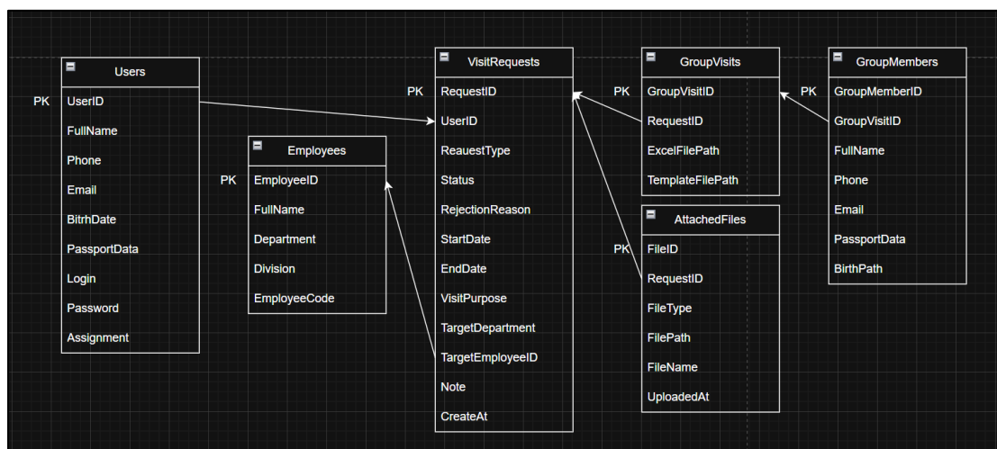
Рисунок 4 – ERD-диаграмма
