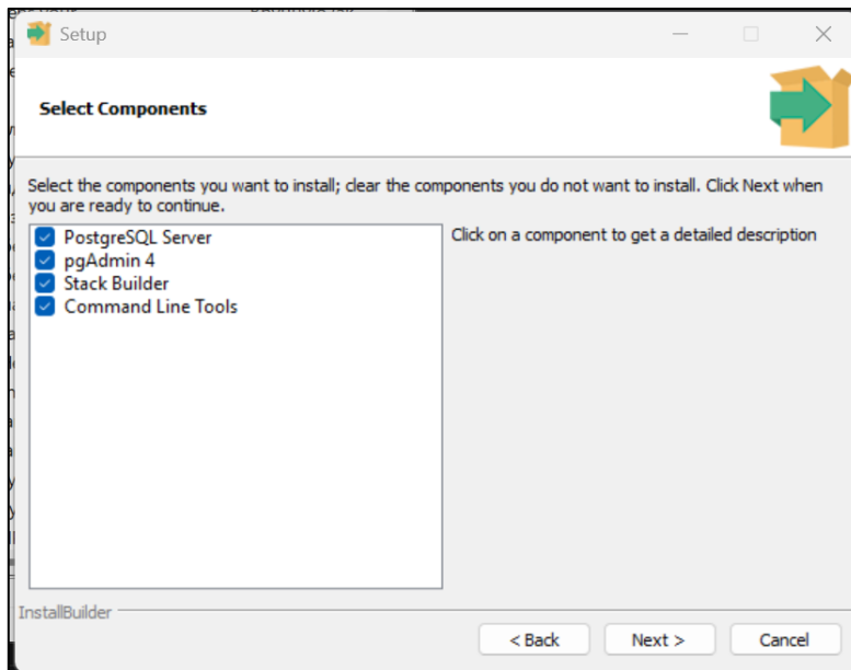
Рисунок 1 – Установка Postgres
